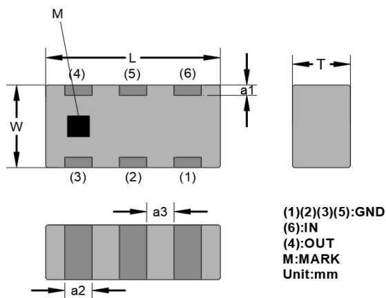
产品外形
