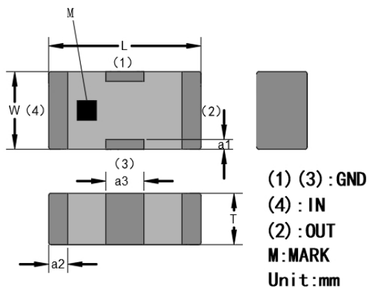
产品外形
